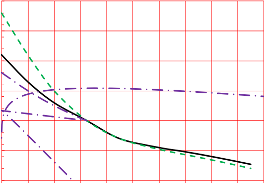
FIG.7: R_{DS(on)} I_{D(on)} V_{GS}
